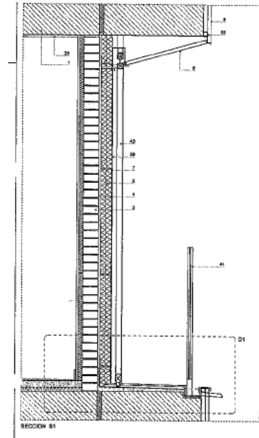
Sección constructiva fachada Sur
