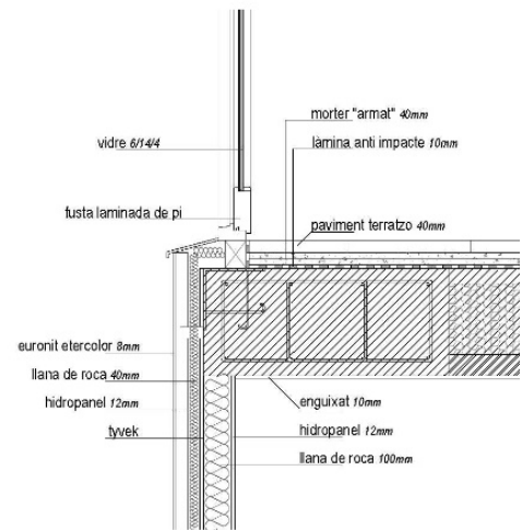
Detalle constructivo ventanas
