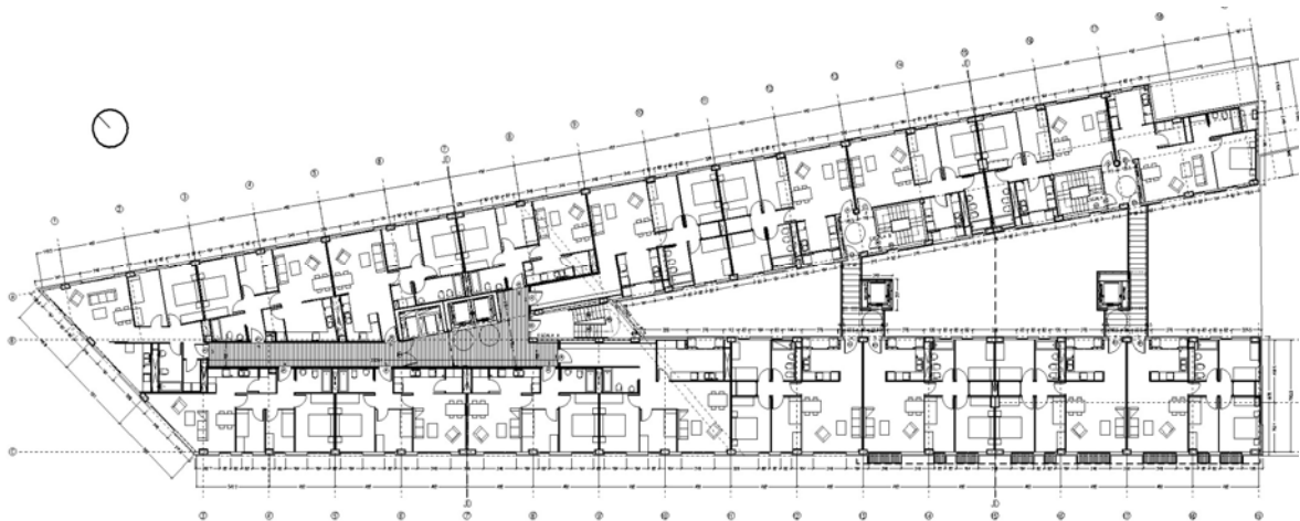
Planta de distribución tipo.
