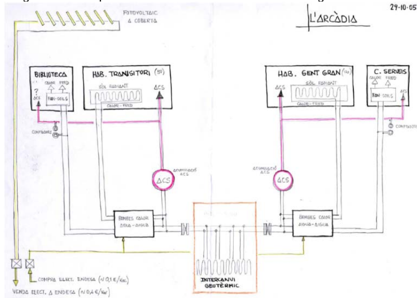
Esquema de funcionamiento de las instalaciones térmicas del edificio.
