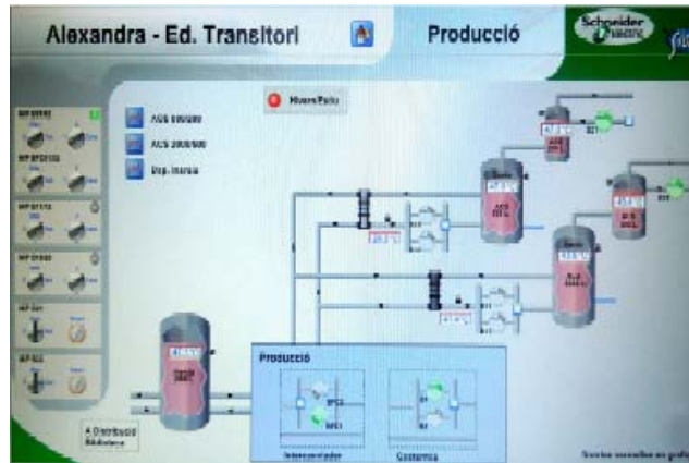
Monitorización y control telemático.
