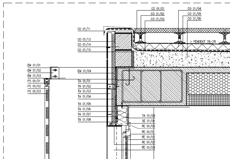
Detalle constructivo cubierta.
