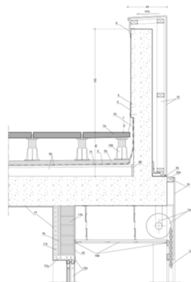
Cubierta en fase de ejecución y sección constructiva.
