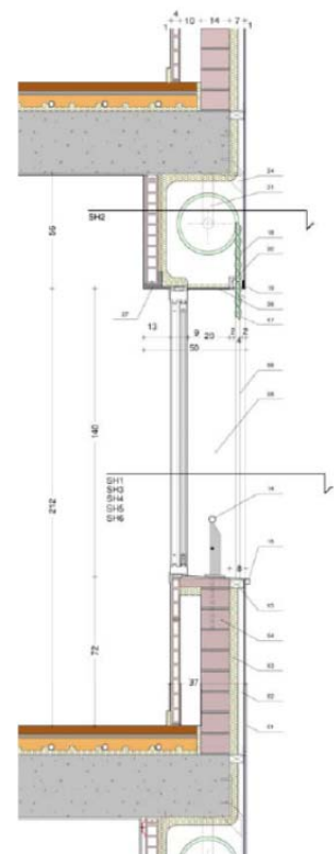
Ventana acabada con las persianas enrollables de lama orientable motorizadas y sección de la fachada por la ventana.
